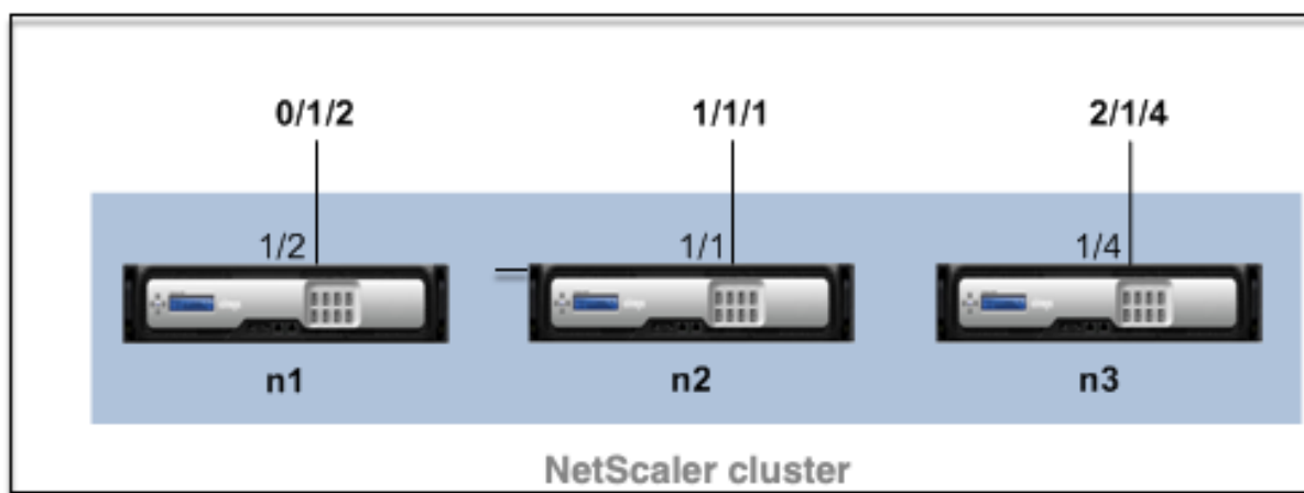
Abbildung 1. Benennungskonvention für Schnittstellen in einem Cluster
