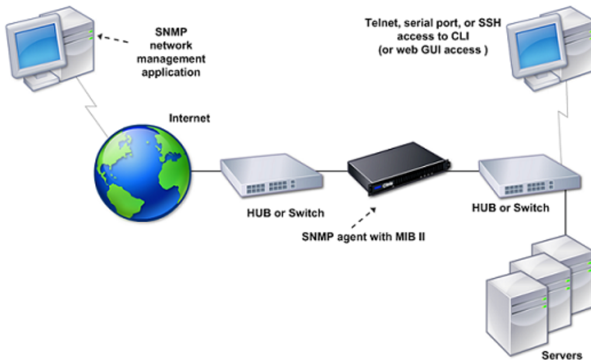
Abbildung 1. SNMP auf der NetScaler-Appliance
