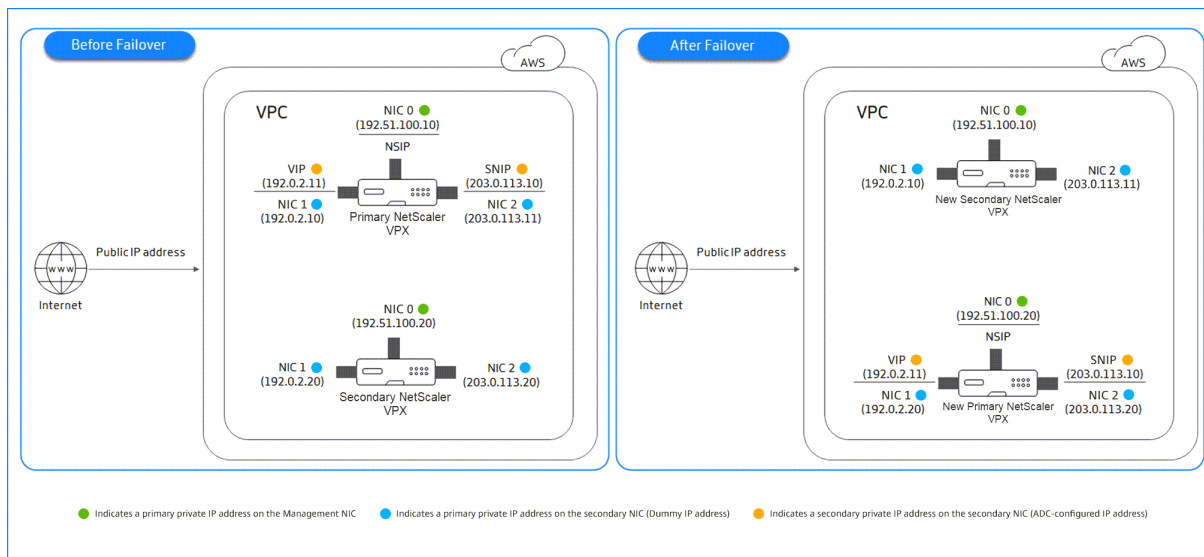
Abbildung 1. Ein NetScaler VPX HA-Paar auf AWS mit privater IP-Migration
