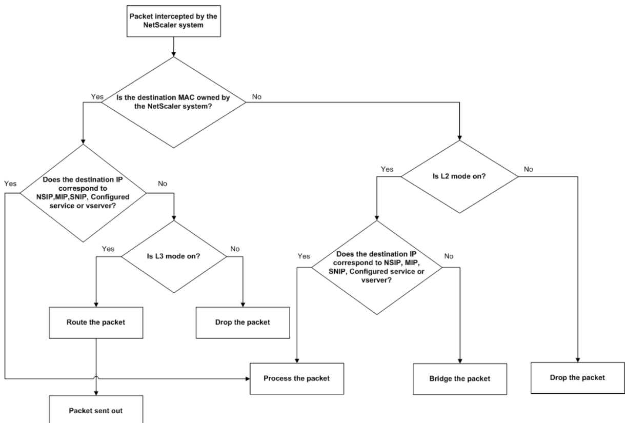
Abbildung 1. Interaktion zwischen Layer-2- und Layer-3-Modi
