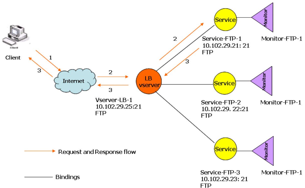
Abbildung 2. Lastenausgleich FTP-Server-Entitätsmodell
