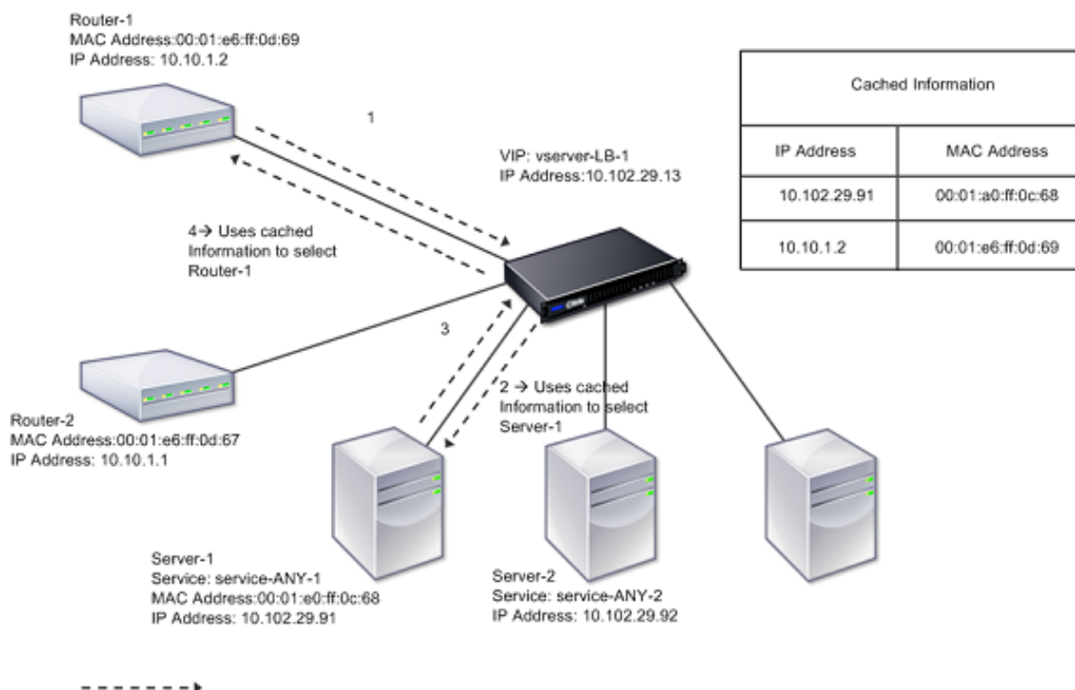
Abbildung 1. MAC-basierten Weiterleitungsmodus
