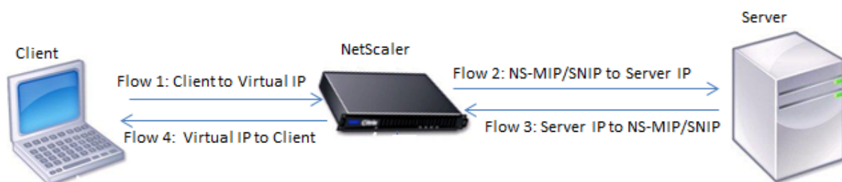
Abbildung 1. NetScaler-Flowsequenz
