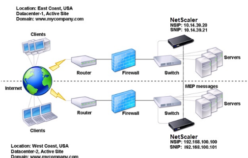
Abbildung 1. Grundlegende GSLB-Topologie
