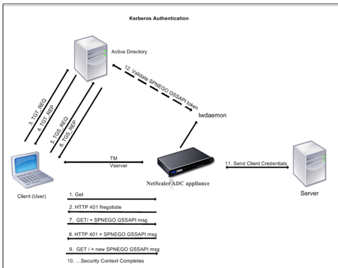
Abbildung 1. Kerberos-Authentifizierungsprozess auf NetScaler
