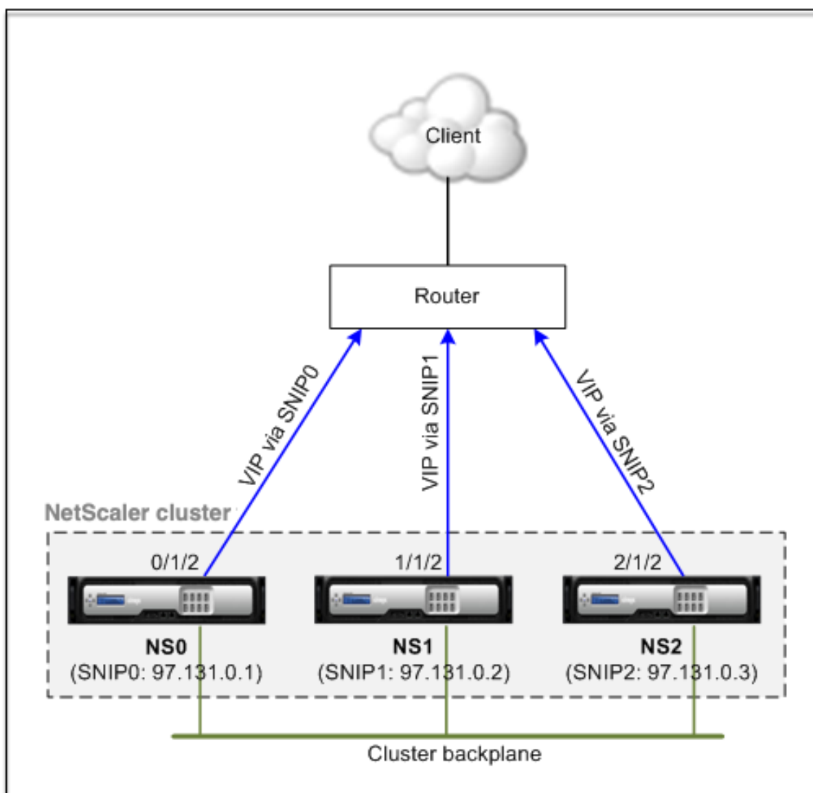
Abbildung 1. ECMP-Topologie
