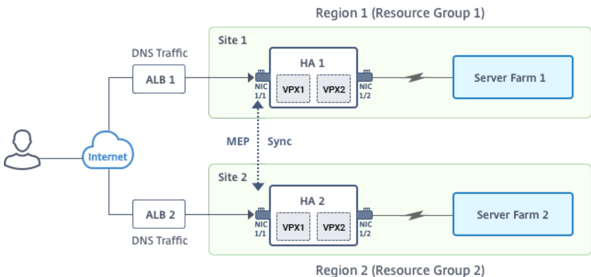
Abbildung: GSLB auf Active-Standy HA-Bereitstellung in Azure
