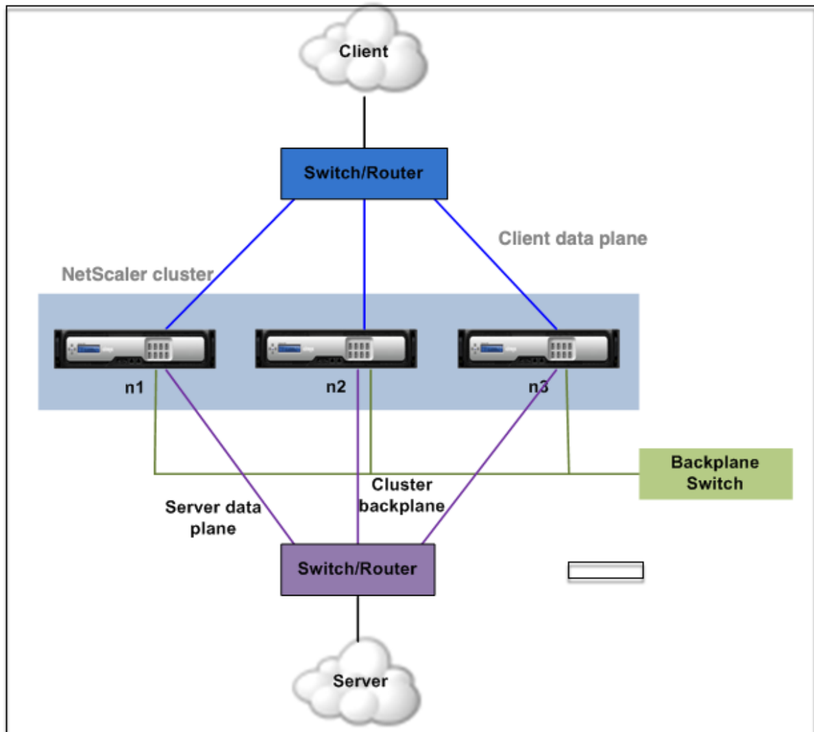
Abbildung 2. Cluster-Kommunikationsschnittstellen - L2-Cluster
