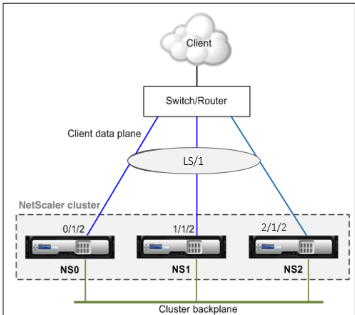
Abbildung 2. Verkehrsverteilungsfluss mit Linksets
