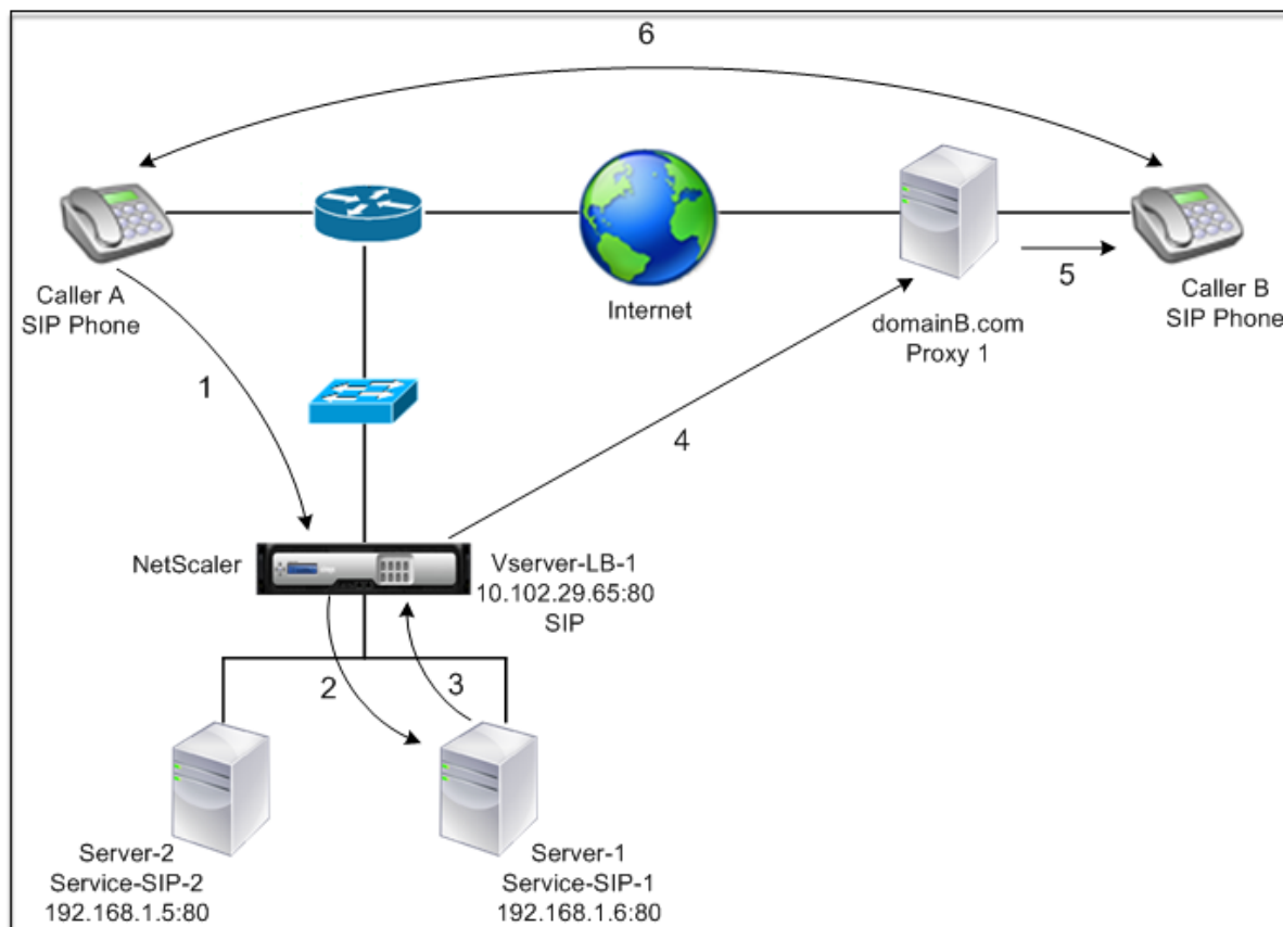
Abbildung 2. SIP Load Balancing Topologie
