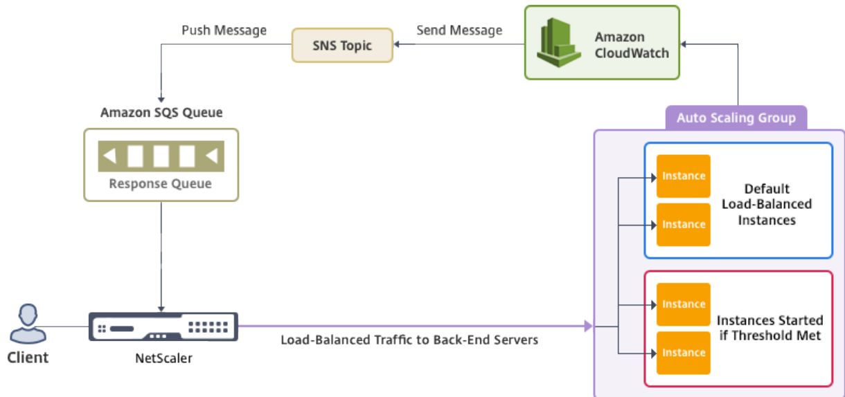
Diagramm: AWS Autoscaling-Service mit einer NetScaler VPX-Instanz
