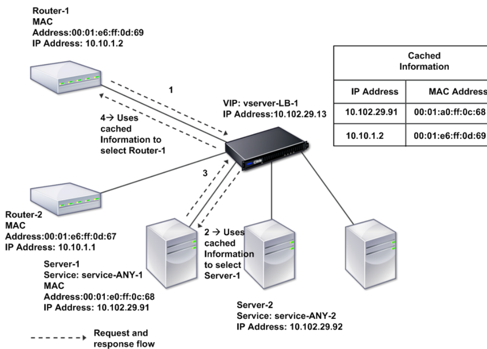
Abbildung 2. Mac-basierter Weiterleitungsprozess
