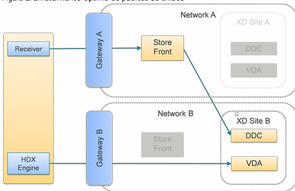
Figura 2. Enrutamiento óptimo de puertas de enlace
