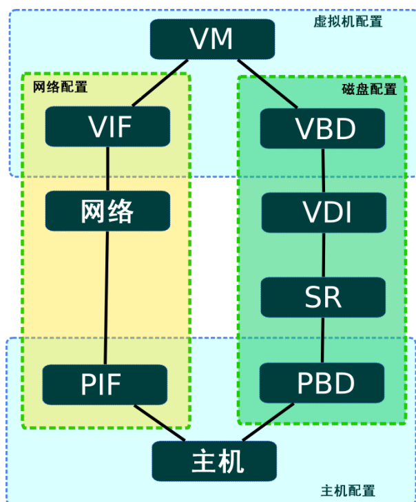
管理 VM、主机、存储和网络的 API 类的图表概述
