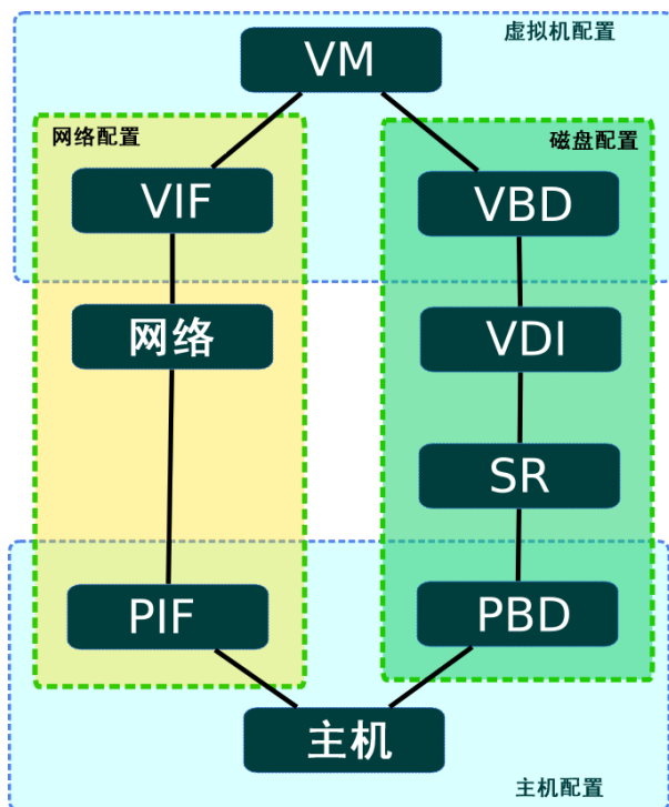
图 3.1. 常见 API 类
