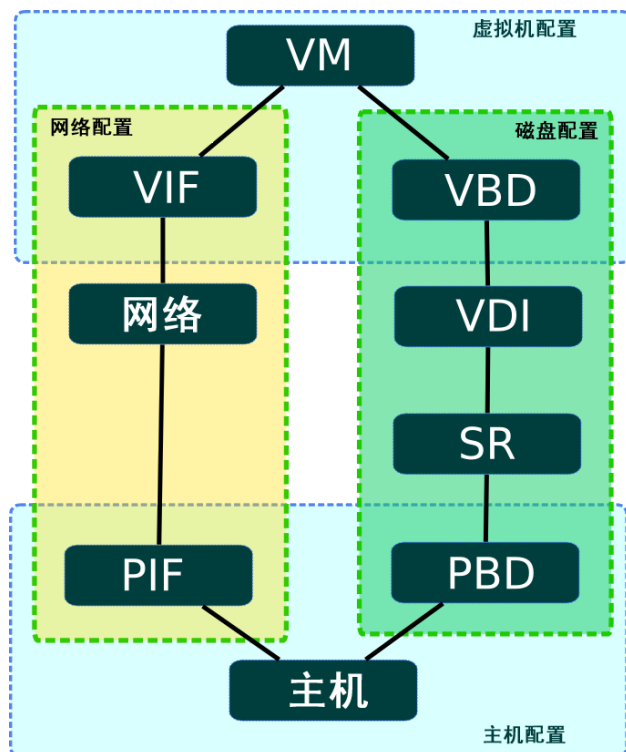
图 3.1. 常见 API 类:
